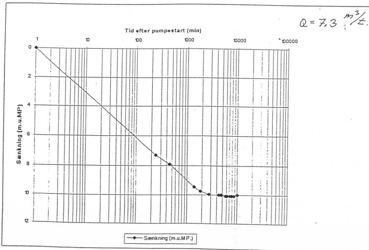
Figur 4.11: Sænkning som funktion af tiden i et semilogaritmsk diagram for boringen ved Jacobsminde.
