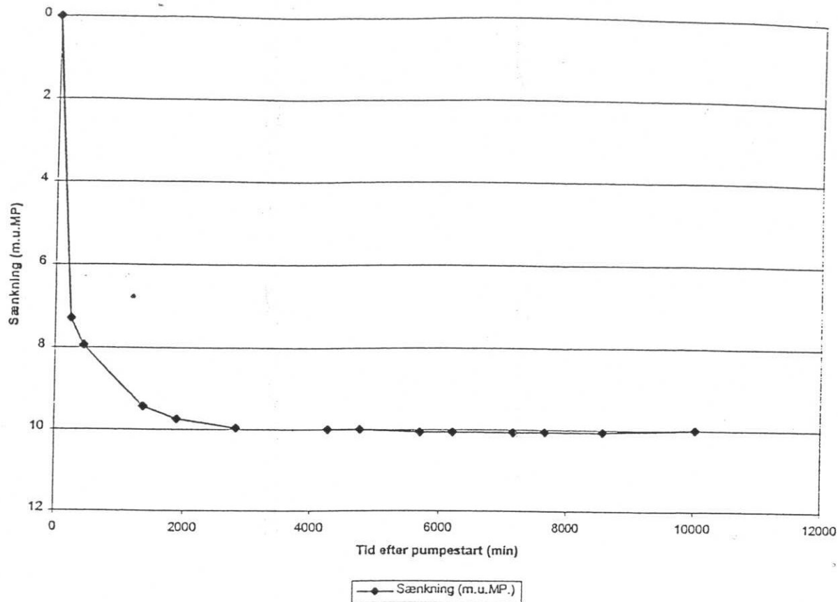
Figur 4.10: Observeret sænkning i boringen ved Jacobsminde med en ydelse på ca. 7.3 m 3 /h.
