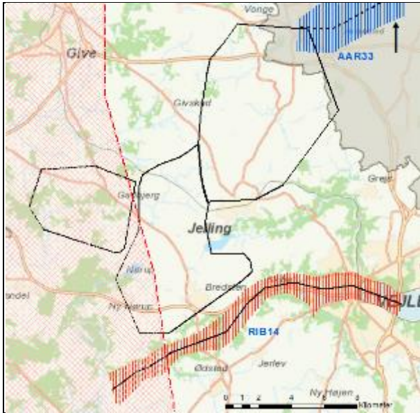
Kort over en svagt dokumenteret delvist begravet dal (AAR33) i Indsatsområde Hvejsel og en veldokumenteret delvist begravet dal (RIB14) syd for kortlægningsområdet (GEUS 2009) samt den østlige afgrænsning af Brande Graven
