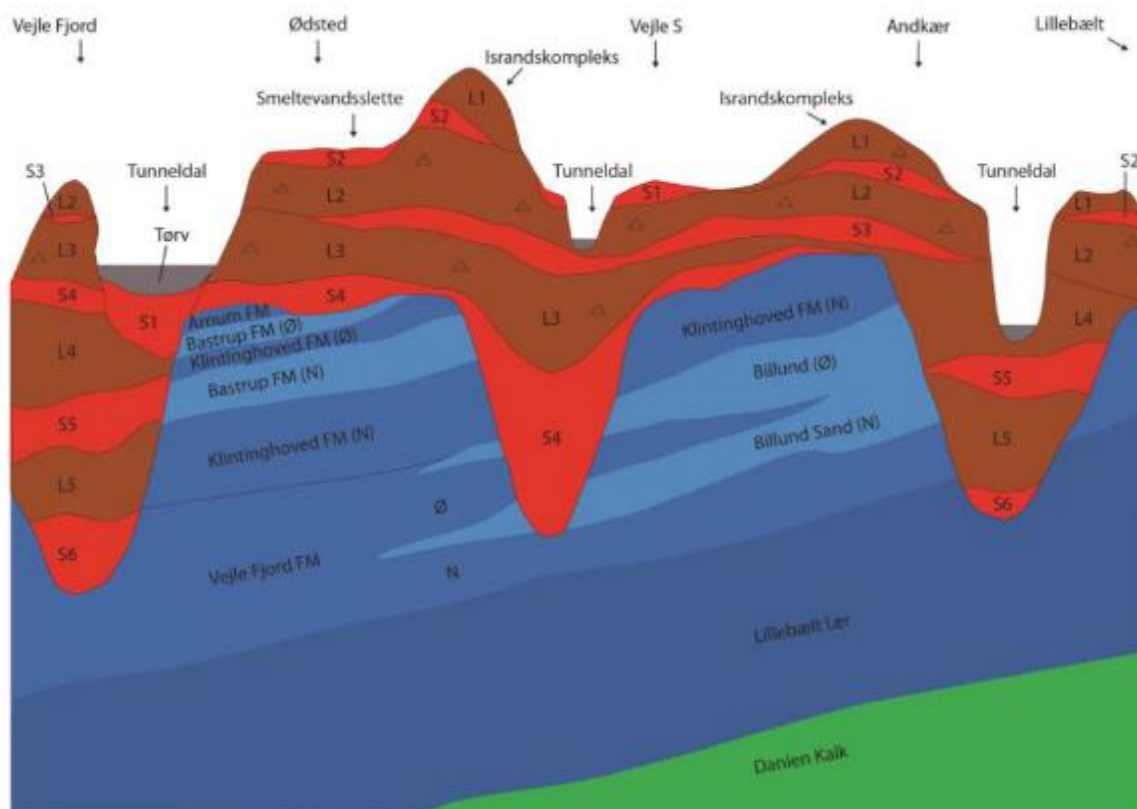
Geologisk profil (forsimplt tænkt profil som viser alle modellag og geologiske strukturer) fra Lillebælt med tunneldal nord for Brejning, over Andkær til Vejle Syd med tunneldal ved Mølholmdalen. Mellem Andkær og Vejle Syd samt Vejle Syd og Ødsted ses israndskomplekser (vidnesbyrd om at her har isen stået, israndslinjer). Ved Ødsted ses en smeltevandsslette som er opstået ved, at isranden er begyndt at trække sig tilbage (smelte) og store mængder sedimenter er skyllet ud foran og har dannet sletten. Længst mod vest ses den største tunneldal, Vejle Fjord
