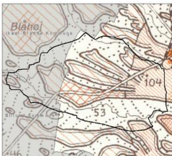
Landskabskortet viser mod øst i modelområdet et morænelandskab fra sidste istid og længere mod vest langstrakte tunger "bakkeøer" med ler- og sandbund og hedesletter fra næstsidste istid (Per Smed 1980)
