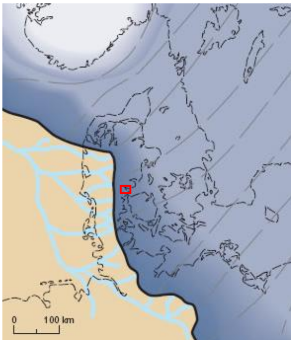
Isens største udbredelse i sidste istid Weichsel Den røde boks viser kortlægningsområdet (M.Houmark-Nielsen & K.H.Kjær, 2005).
