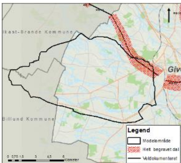
Kort over begravet dal (RIB 15) i modelområdet (GEUS 2009)
